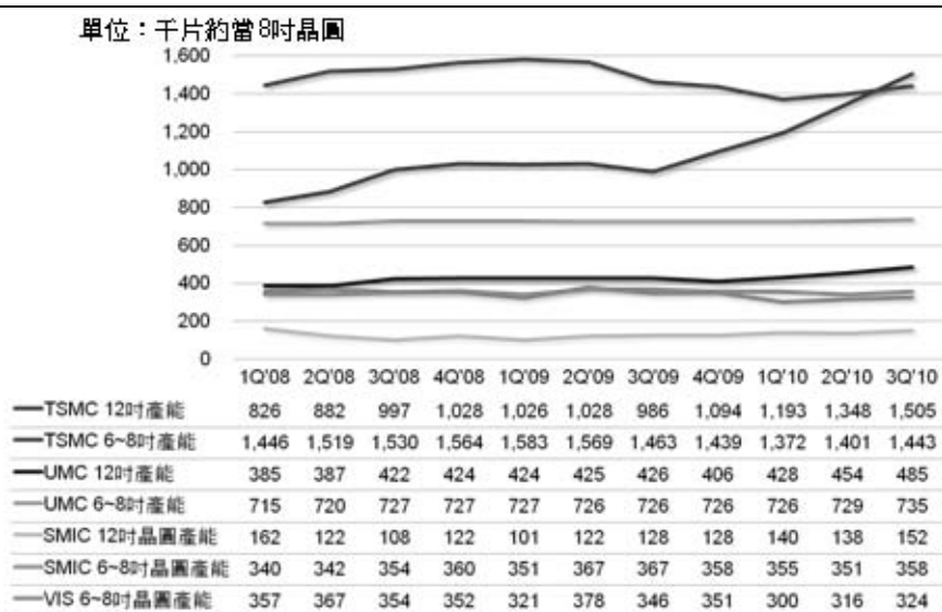
1Q'08~3Q'10 大中華地區前 4 大晶圓代工業者 12 吋及 6~8 吋晶圓產能變化
